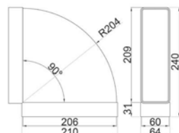
WYMIARY [MM]
