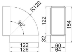
WYMIARY [MM]
