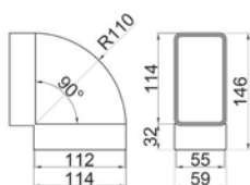
WYMIARY [MM]
