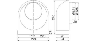
WYMIARY [MM]
