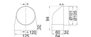
WYMIARY [MM]
