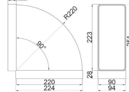
WYMIARY [MM]
