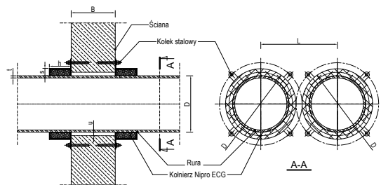
Rys. Przejście rur palnych przez ścianę zabezpieczone kołnierzem Nipro ECG.
