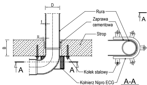
Rys. Przejście rury palnej przez strop z kołnierzem Nipro ECG w kształcie U umieszczonym na kolanie rury.
